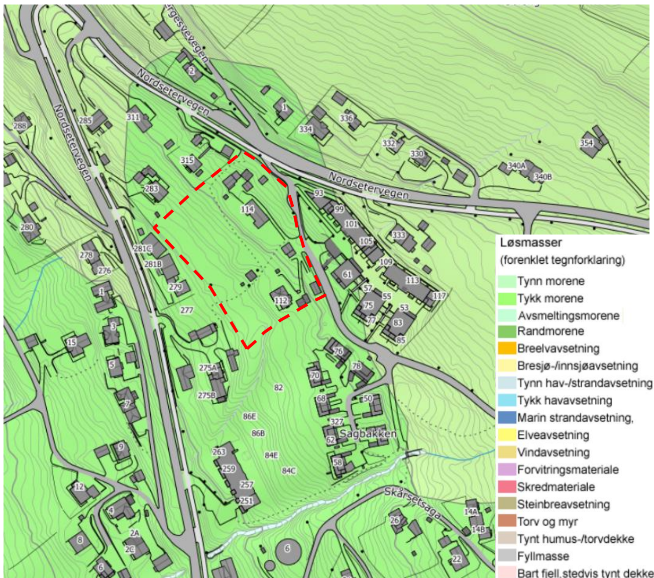
Figur 7 Løsmassekart (NGU, 2021) for reguleringsområdet. Ca. plassering av reguleringsområdet er markert med rødt.
