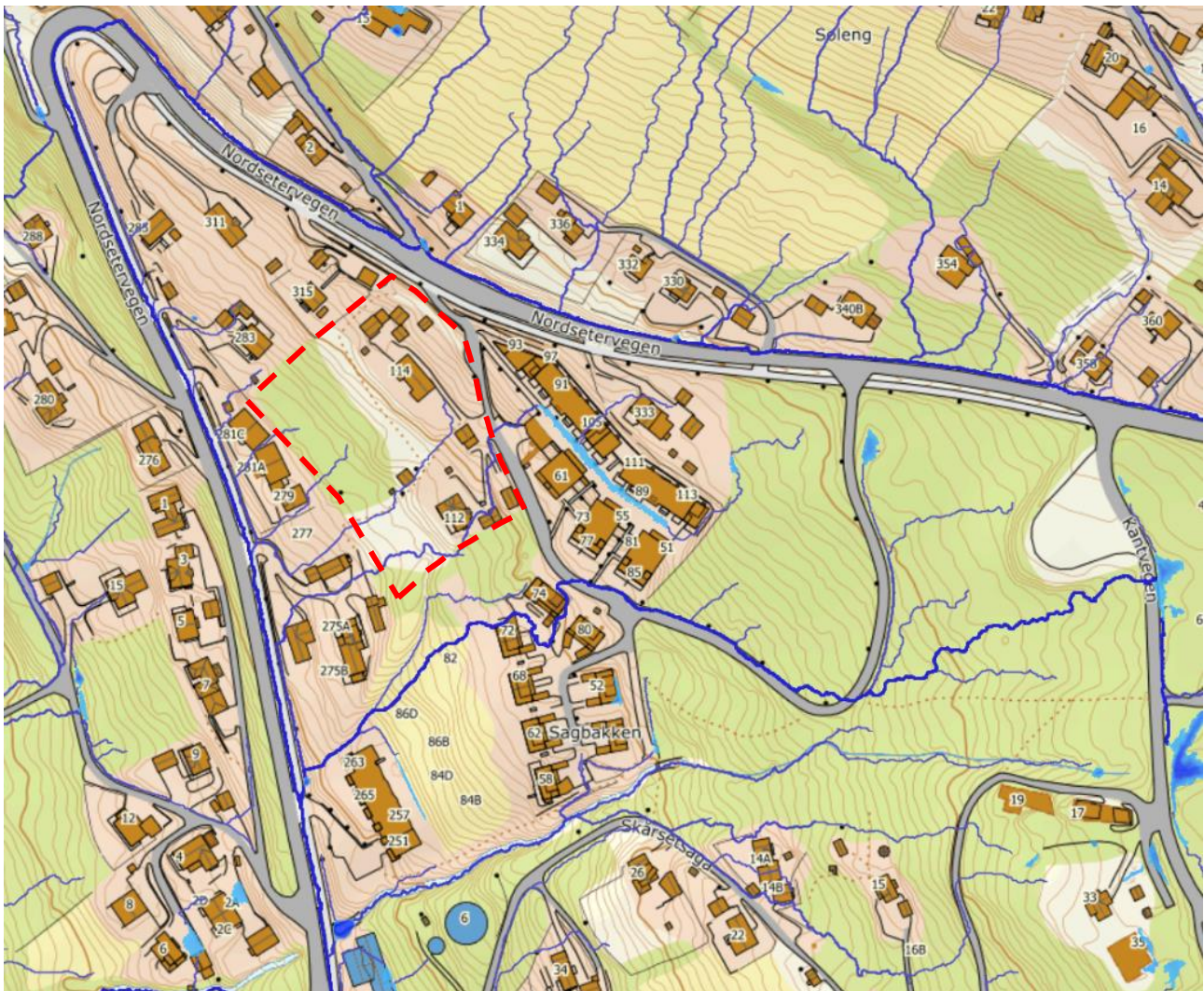
Figur 5 Flomveiskart fra Scalgo med grunnlag fra laserdata (2019) med oppløsning på 0.25 m. Ca. plassering av reguleringsområdet er markert med rødt.
